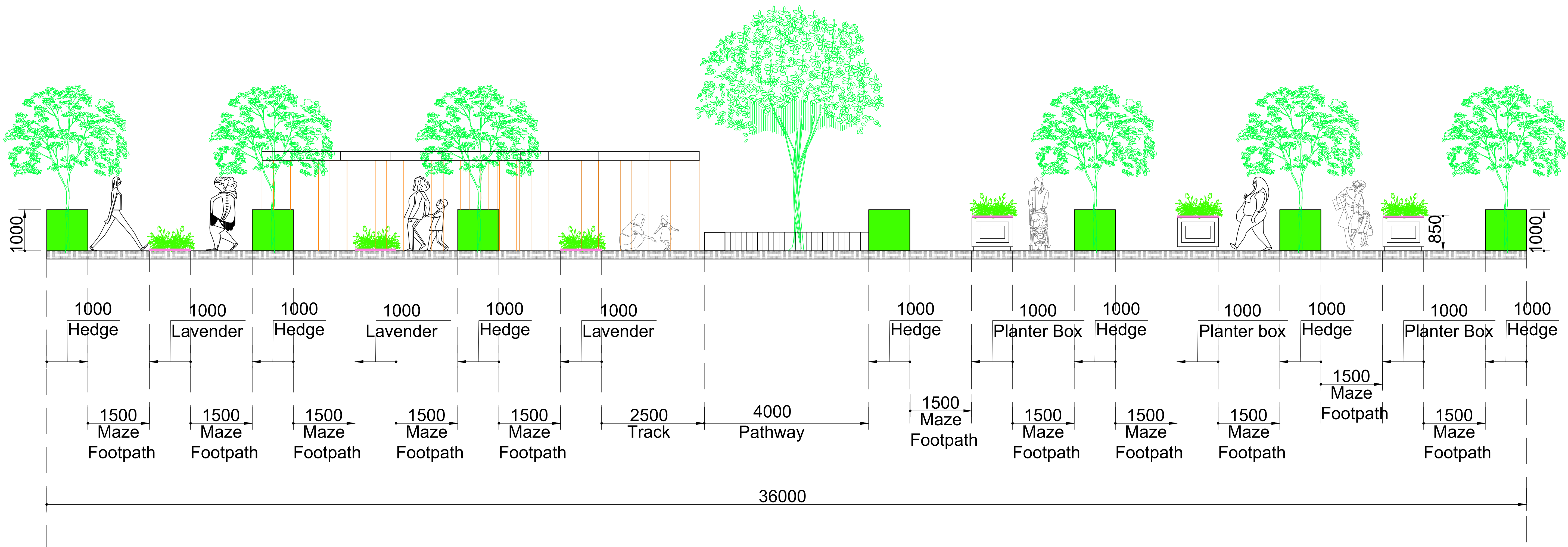
1 SECTION A-A 1:50 @ A1 / 1:100 @ A3
