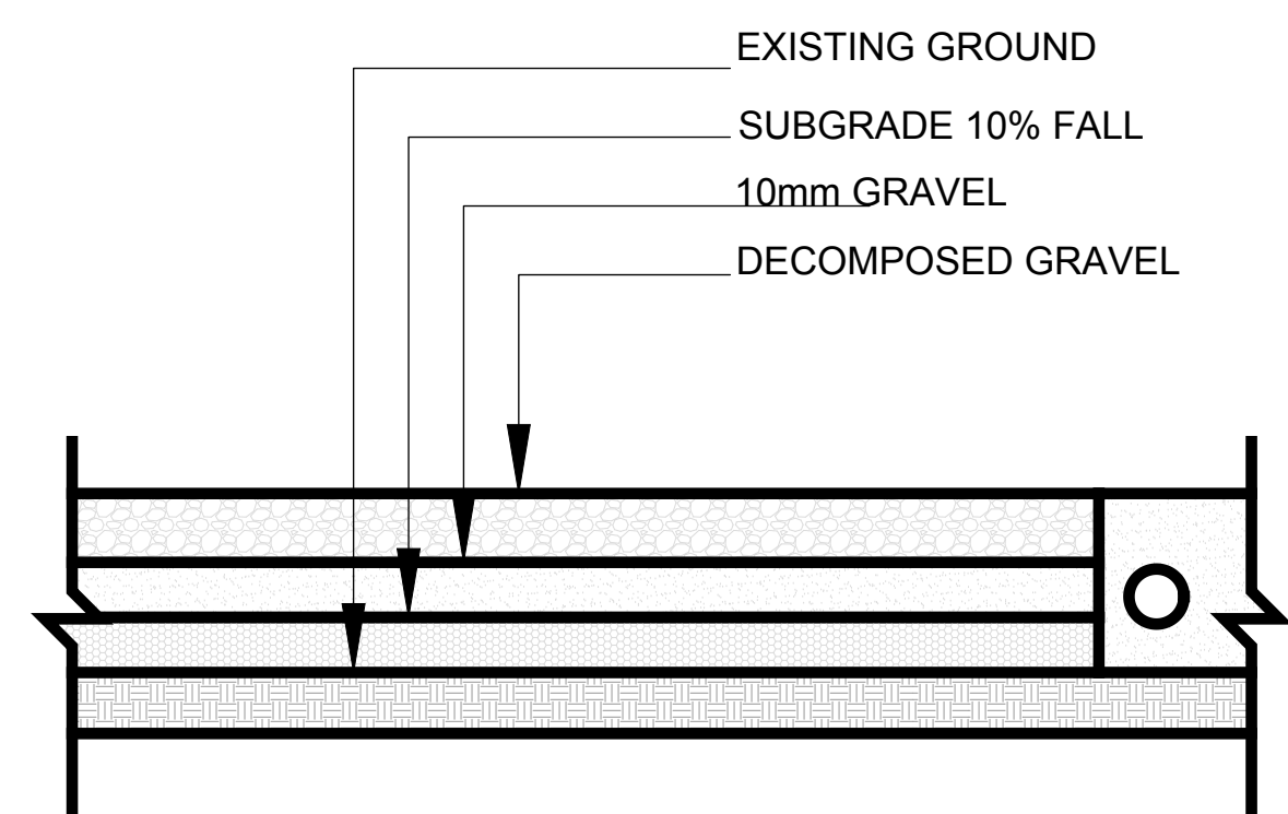
1 SECTION A-A 1:50 @ A1 / 1:100 @ A3
